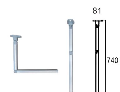
GR-ZT503 テーブルレッグ (中折れ) US020052 Size:740 (388+232) *40mm
