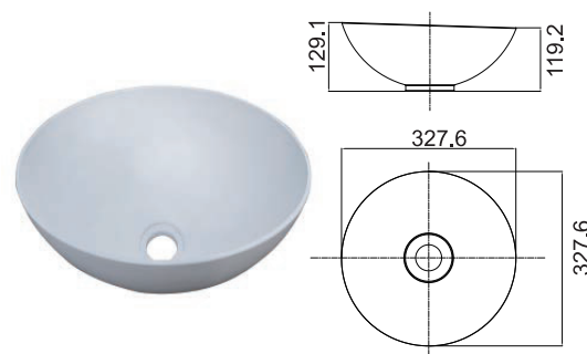
GR-TP05 丸型アクリルシンク・小 US020041 Size: 327.6*327.6*119.2/129.1mm Thick: 5mm
