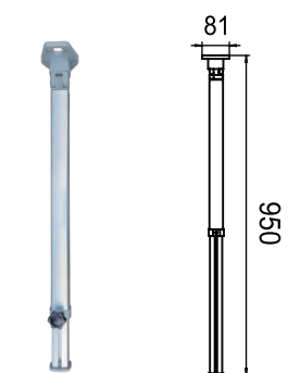
GR-ZT505 テーブルレッグ伸縮式 US020053 Size: (652-950) *40mm
