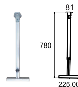
GR-ZT501 テーブルレッグ伸縮式 US020050 Size:555-780*225/40mm
